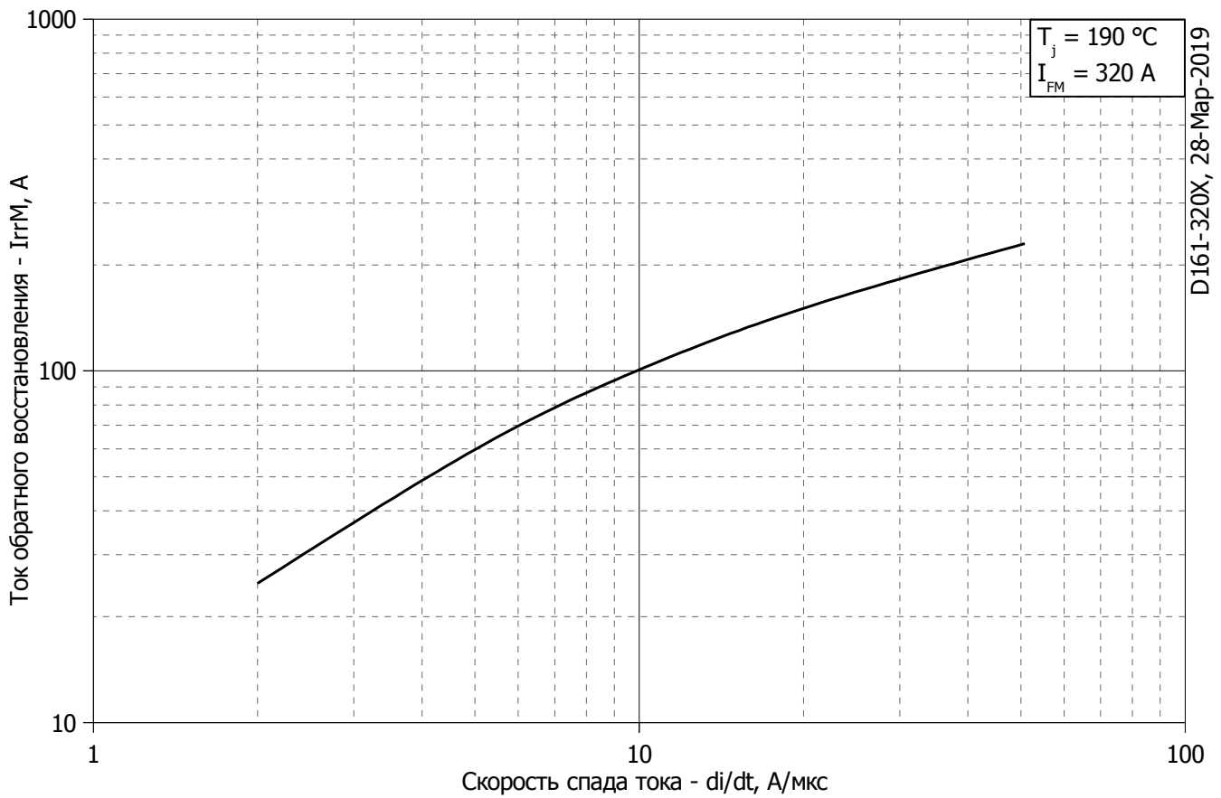
Рис. 5 – Зависимость максимального тока обратного восстановления I_{TRM} от скорости спада прямого тока di_R/dt
