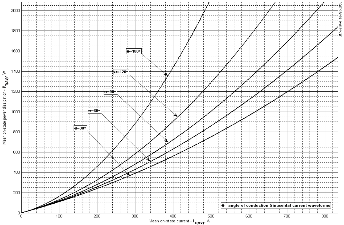
Рис. 9 – Зависимость потерь мощности P_{TAV} от среднего прямого тока I_{TAV} синусоидальной формы при различных углах проводимости ( f=50 Гц)
